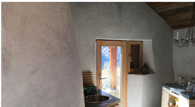
Raboccadüra da chaltschina fatta cun sablun da l'En e chaltschina stüzza da la Val S-charl glischada cun üna chazzöla veneziana, foto Delphine Schmid
